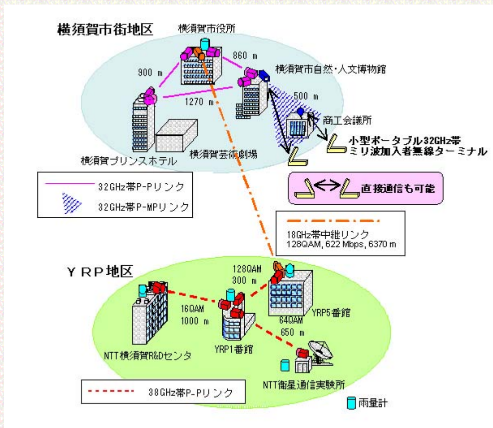
図2 実験ネットワーク全体配置図 (通信品質の変動と降雨量との関係を解析するため随所に雨量計を設置しています)
