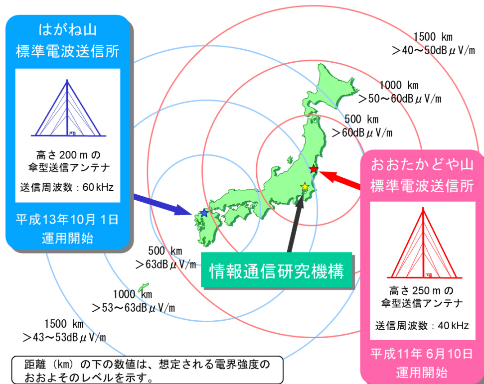
図1 送信所の位置と標準電波（地上波）の推定電界強度
