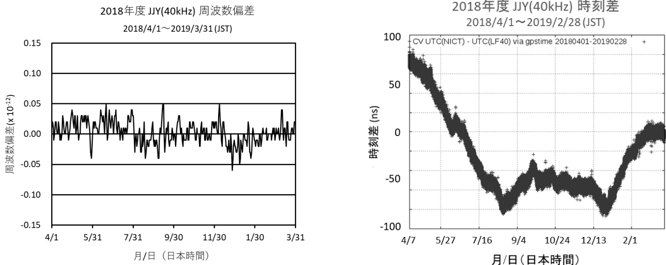
図7 おおたかどや山送信所の周波数偏差と時刻精度 (2018年度)
