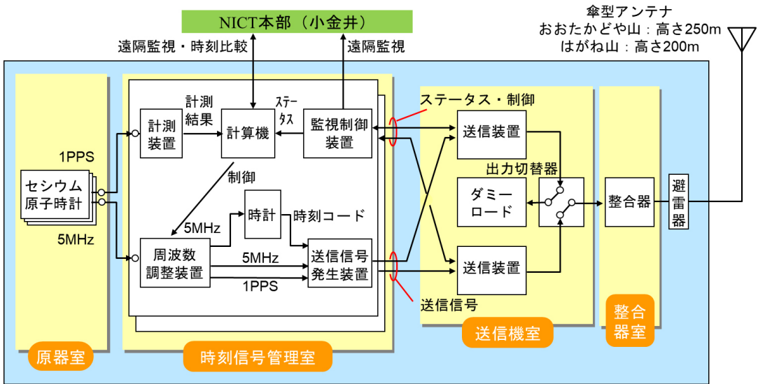
図 2 標準電波発生設備と送信までの構成
