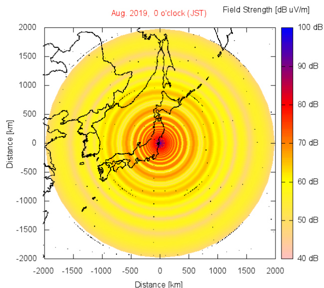
図3 標準電波電界強度予想マップ (2019年8月の0時JST おおたかどや山 40 kHz)
