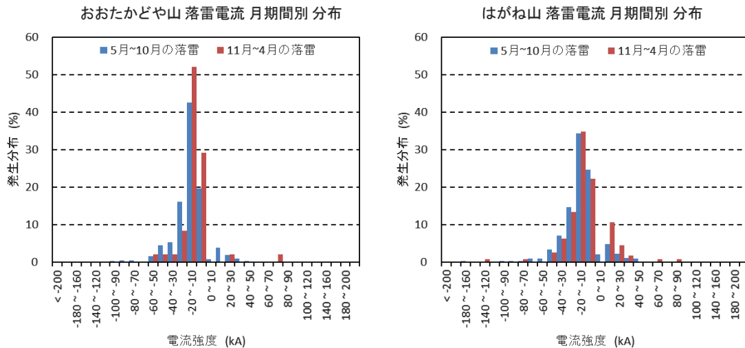
図4 2014年から2018年の各送信所への落雷の電流強度分布 (月期間別)
