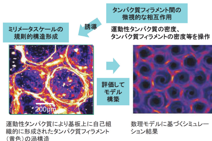
図2 ミクロな生体分子によるマクロな自己組織構造形成
