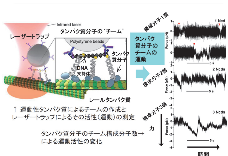
図 1 DNA 支持体-タンパク質分子複合体の作成と活性の計測
