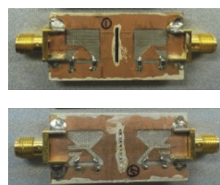
図 8 広帯域アンテナの例
