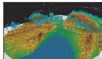
図 5 観測された近畿地方の降雨の 3 次元画像の例
