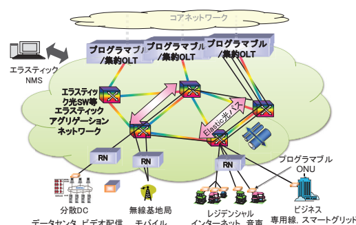
図 6 エラスティック光アグリゲーションネットワークの概要図
