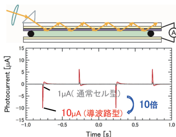
図2 導波路型 bR セルを用いた高効率化
